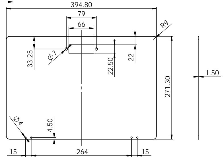
面板尺寸
