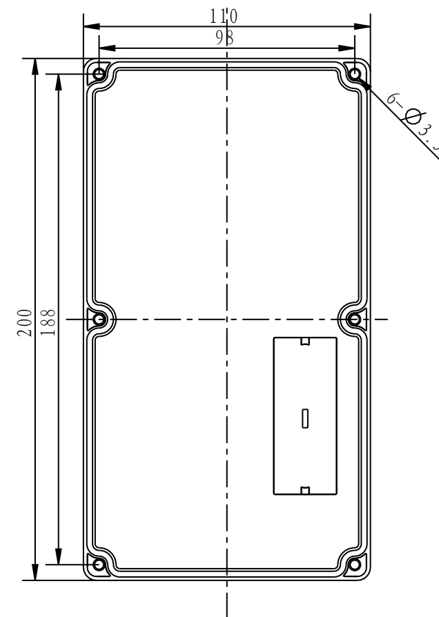
上盖仰视图
