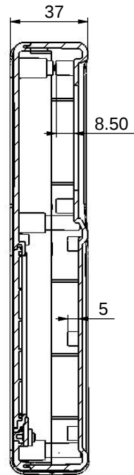
剖面 A-A
