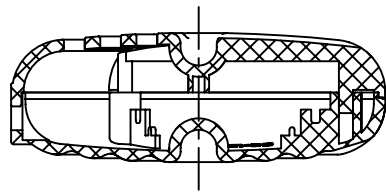
剖面 A-A
