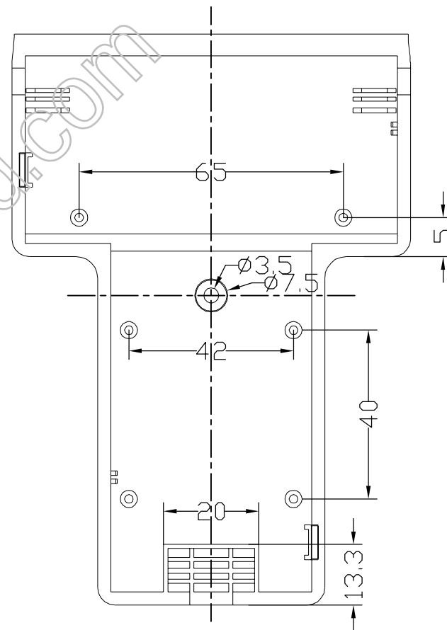
下盖正视图
