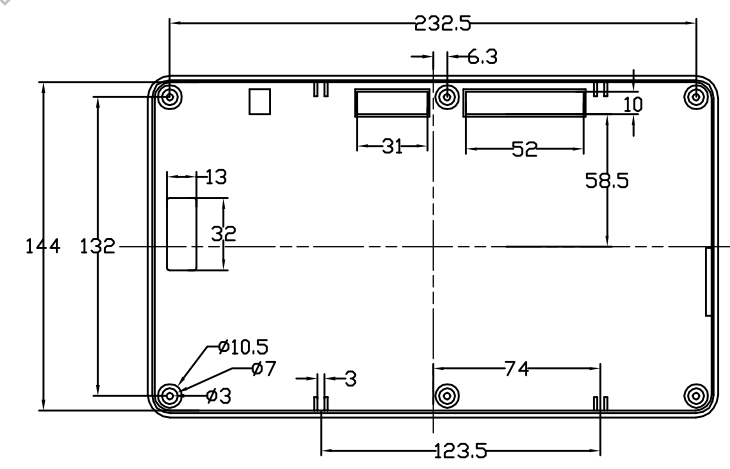
下盖正视图
