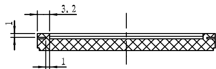
剖面 B-B
