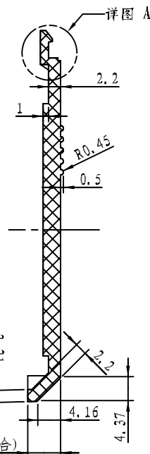
剖面 A-A
