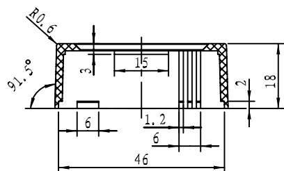
剖面 B-B
