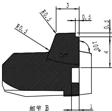
细节 B 比例 5:1
