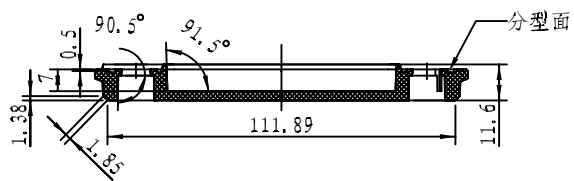
剖面 A-A
