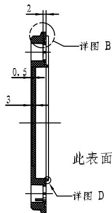
剖面 B-B
