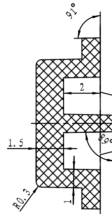
剖面 A-A
