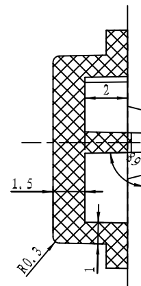
剖面 A-A
