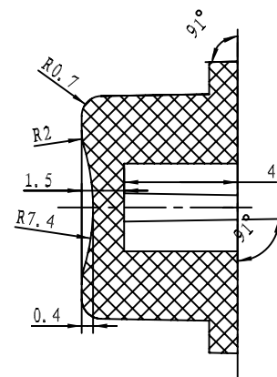
剖面 A-A
