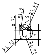
细节 E 比例 1:1
