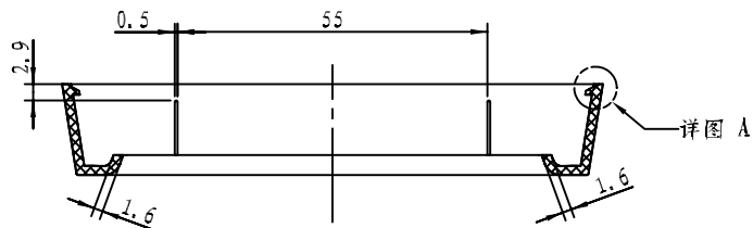
剖面 A-A
