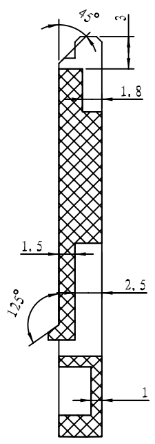
剖面 A-A
