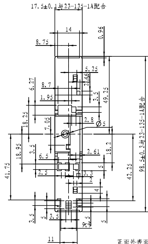
正面外表面
