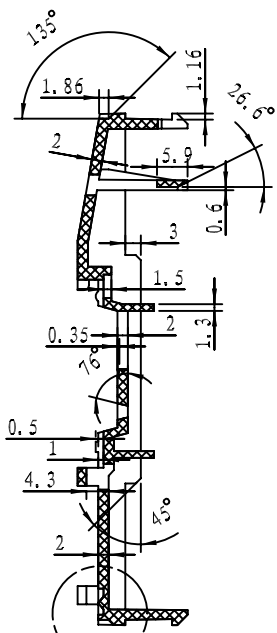
剖面 C-C
