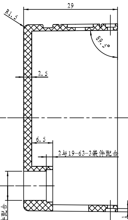
截面 A-A
