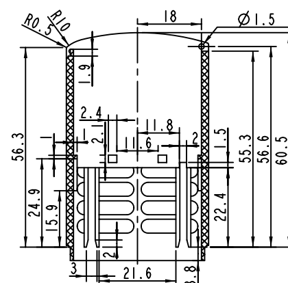
侧面 A-A
