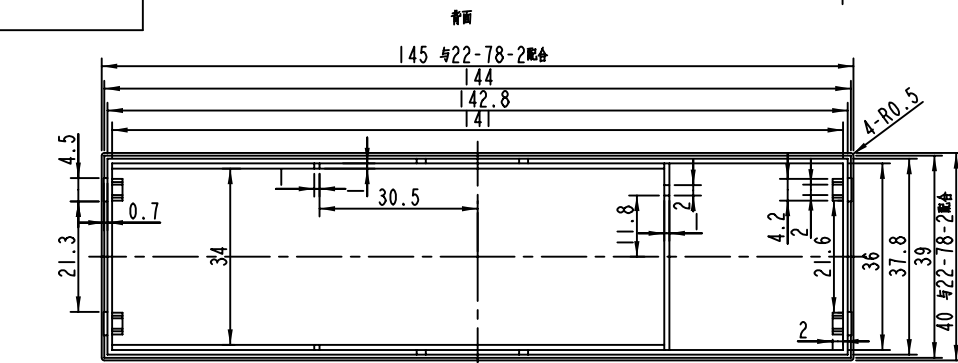
侧面 B-B
