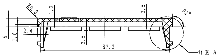
剖面 B-B
