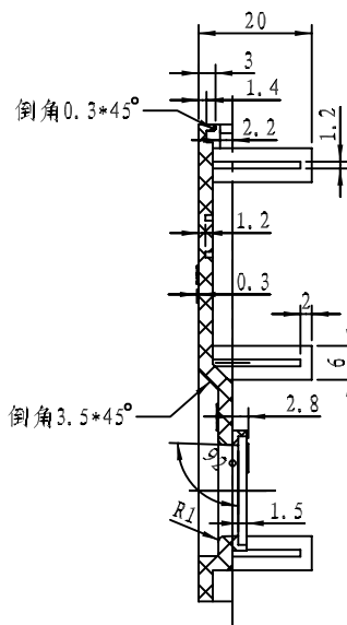
剖面 A-A
