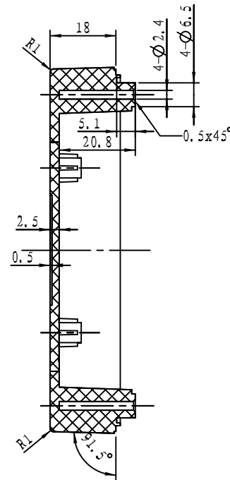
剖面 A-A
