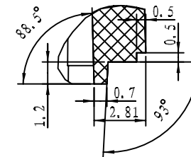
细节 A 比例 5:1
