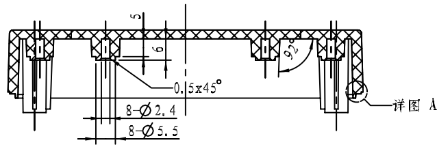
剖面 B-B
