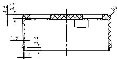
截面 B-B
