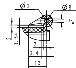
细节 A 比例 1:1
