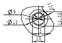
细节 C 比例 1:1
