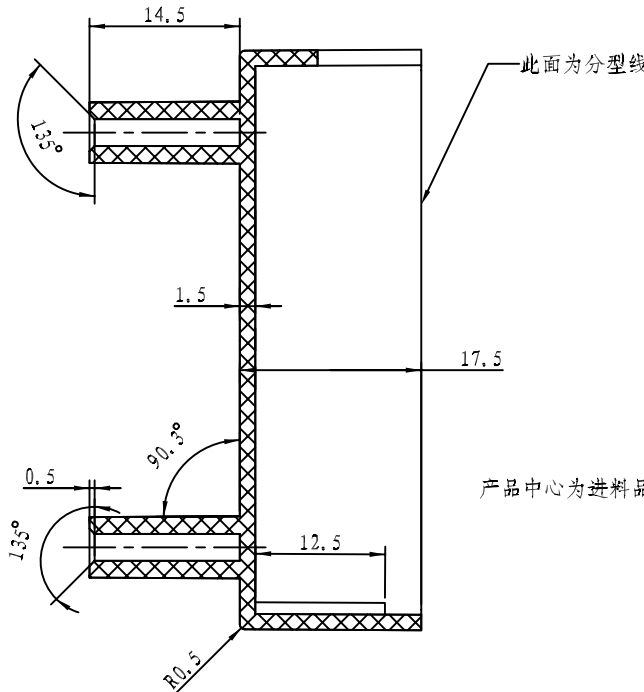
剖面 A-A
