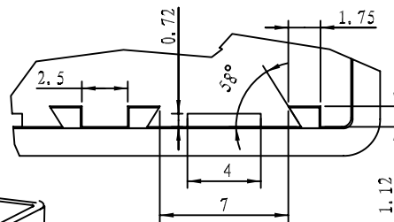
剖面 A-A
