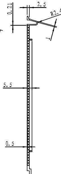
剖面 B-B
