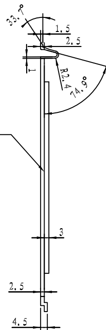
剖面 B-B
