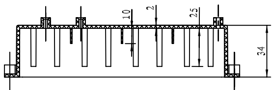
剖面 B-B
