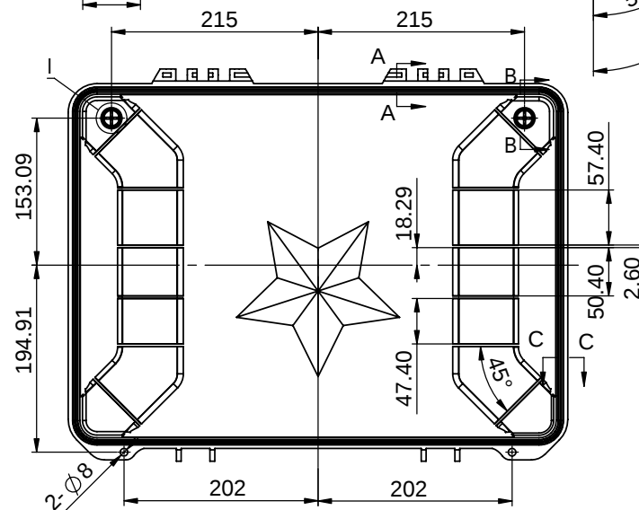
背面（顶杆面）
