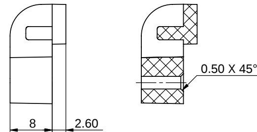
剖面 A-A
