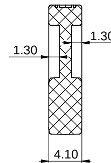
剖面 A-A
