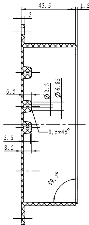
截面 B-B
