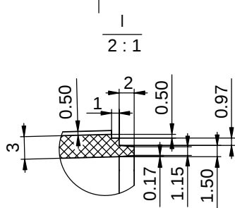
分型面
