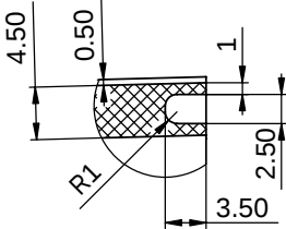
分型面
