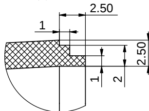
局部视图 B 比例 4:1
