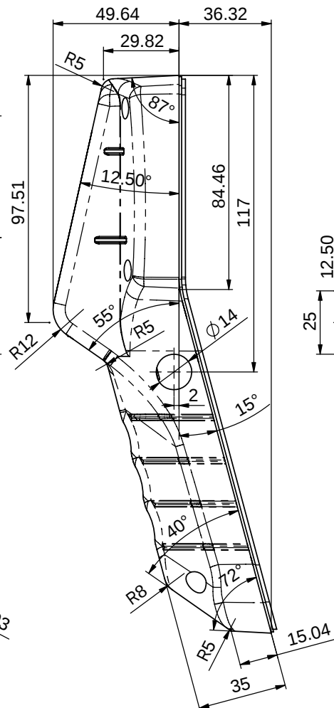
局部视图 B 比例 4:1
