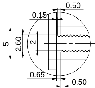
局部视图 D 比例 4:1
