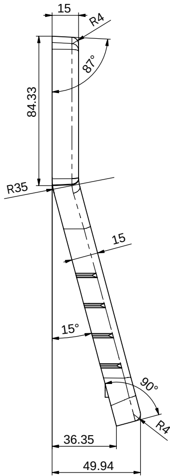
局部视图 D 比例 4:1
