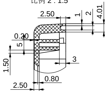
局部视图 B 比例 2:1.5
