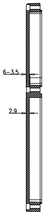
B-B
