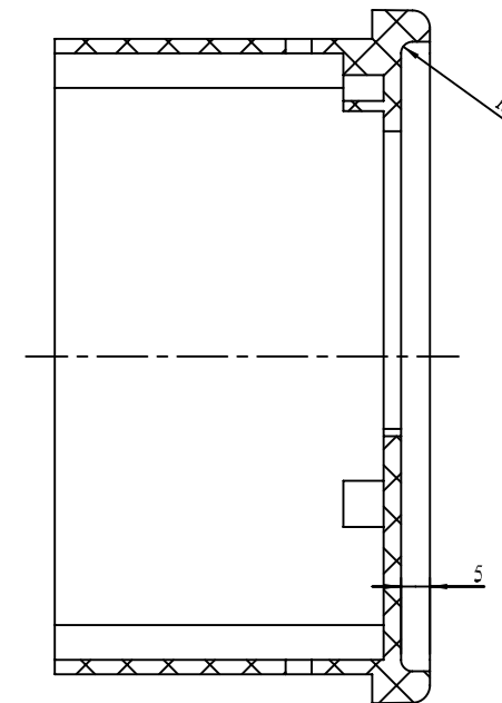
剖面 A-A
