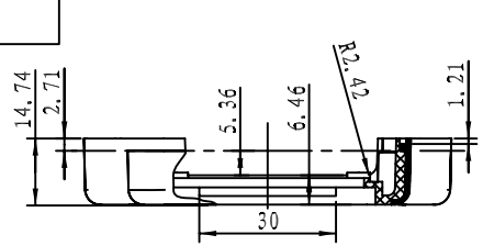
剖面 B-B
