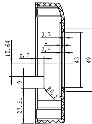
剖面 B-B
