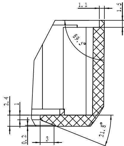
细节 A 比例 3:1
