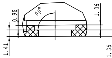
细节 C 比例 3:1
