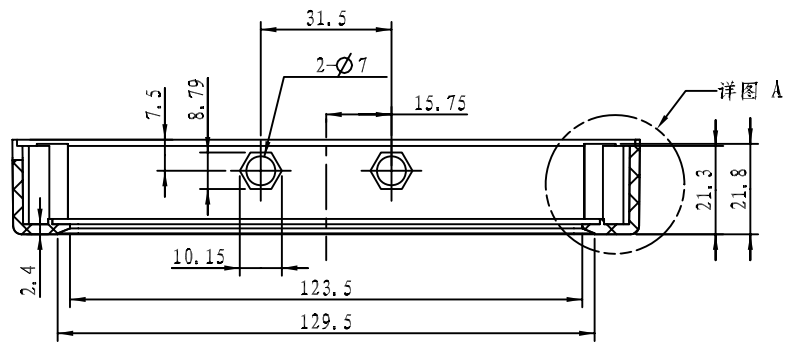
剖面 A-A
