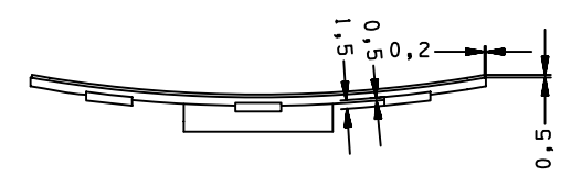
仰视图
