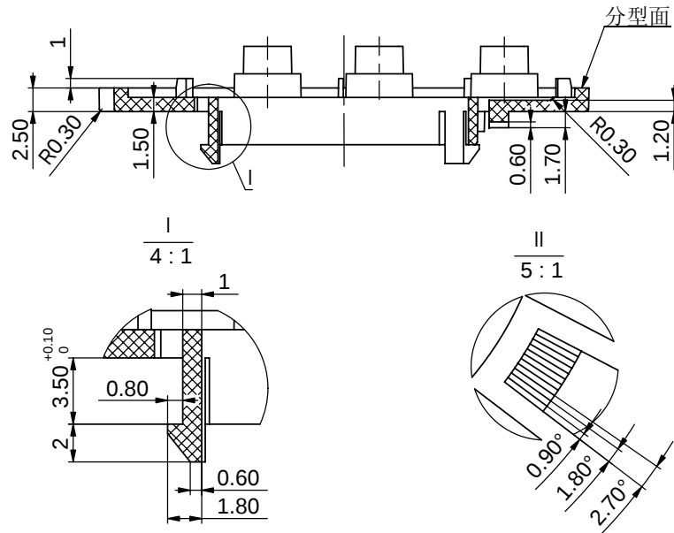
剖面 B-B
