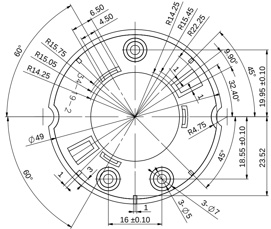
背面(顶杆面)
