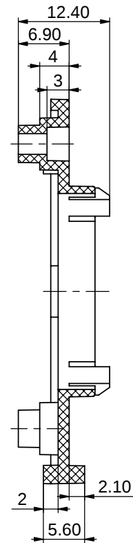
剖面 A-A
