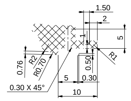
局部视图 E 比例 2.4 : 1
