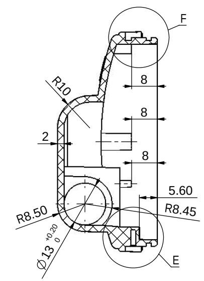
局部视图 F 比例 2.4 : 1
