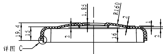
截面 A-A
