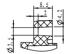
细节 D 刻度 3:2
