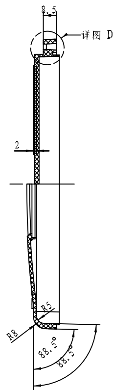
截面 B-B
