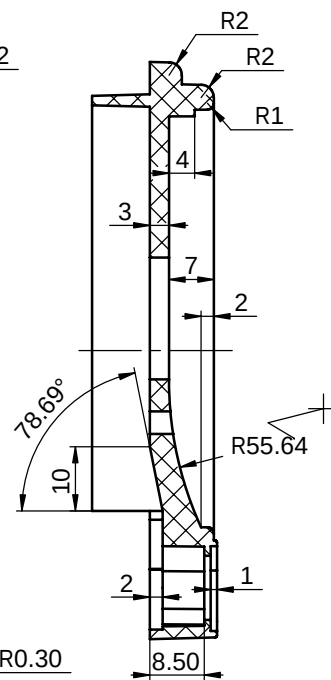
剖面 A-A
