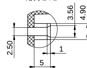
局部视图 E 比例 2:1
