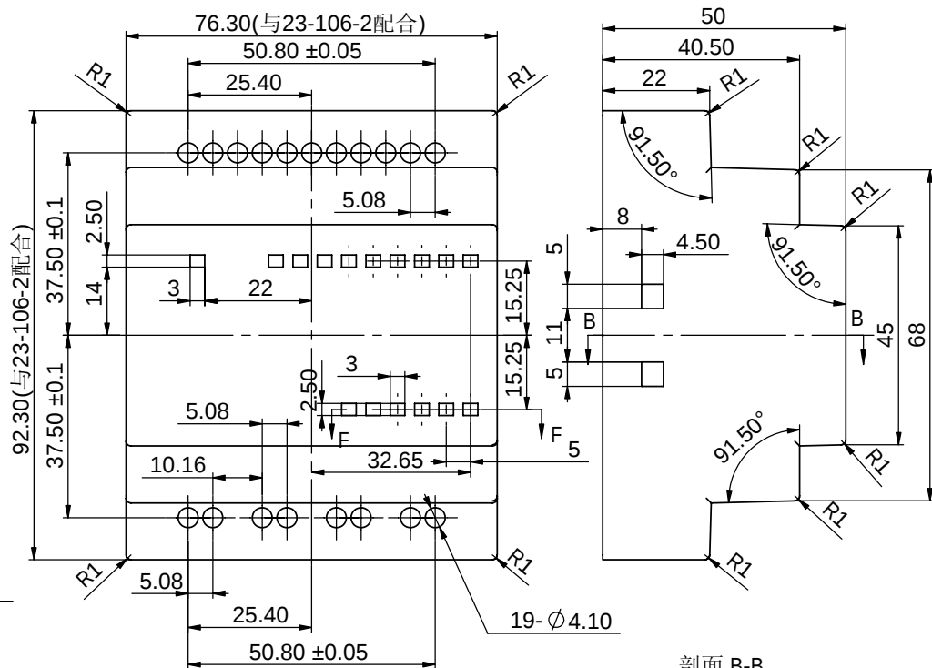
剖面 B-B
