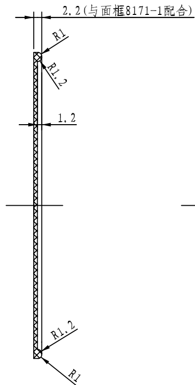
截面 A-A
