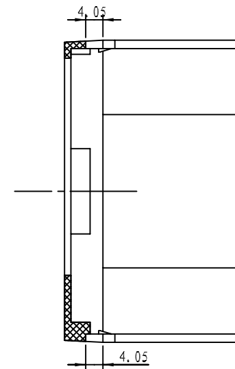
截面 A-A
