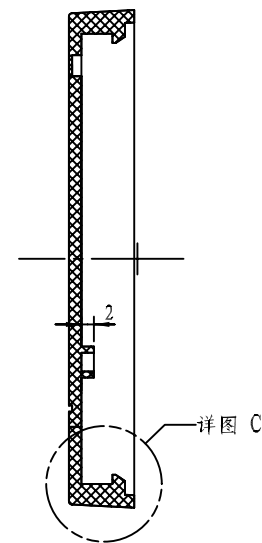
截面 A-A
