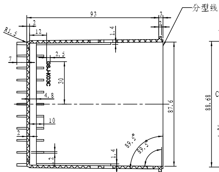
截面 A-A
