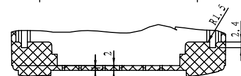
截面 C-C
