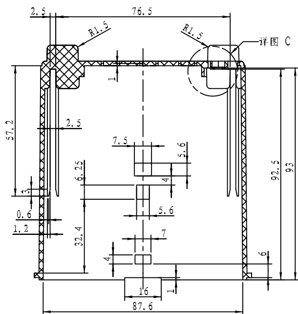
截面 B-B
