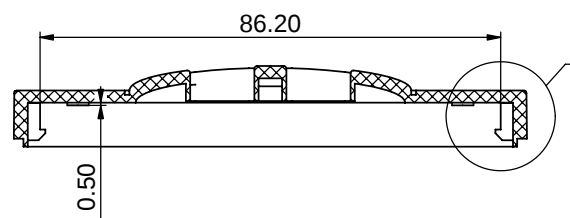
剖面 A-A
