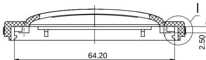
剖面 A-A
