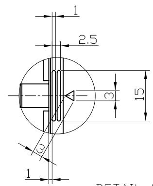
DETAIL H 2 : 1
