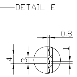
DETAIL F 2 : 1
