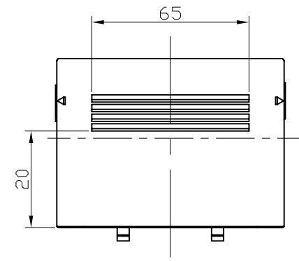
外表面--砂面 DETAIL E 2 : 1
