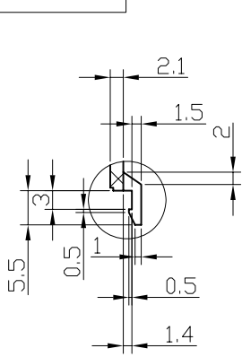
DETAIL G 2 : 1
