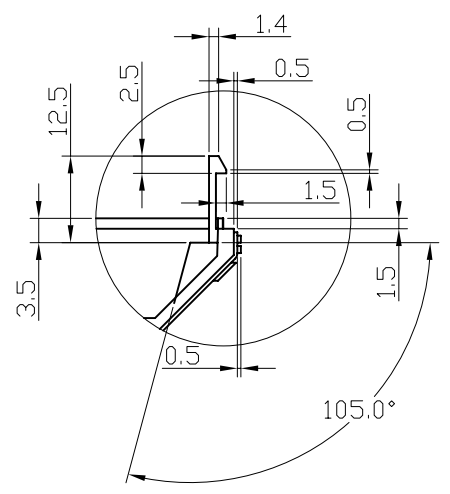
外表面--砂面 DETAIL E 2 : 1
